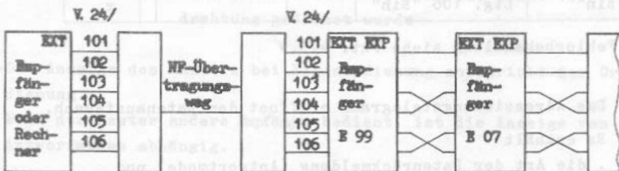
Zusammenschaltung mit Modem
