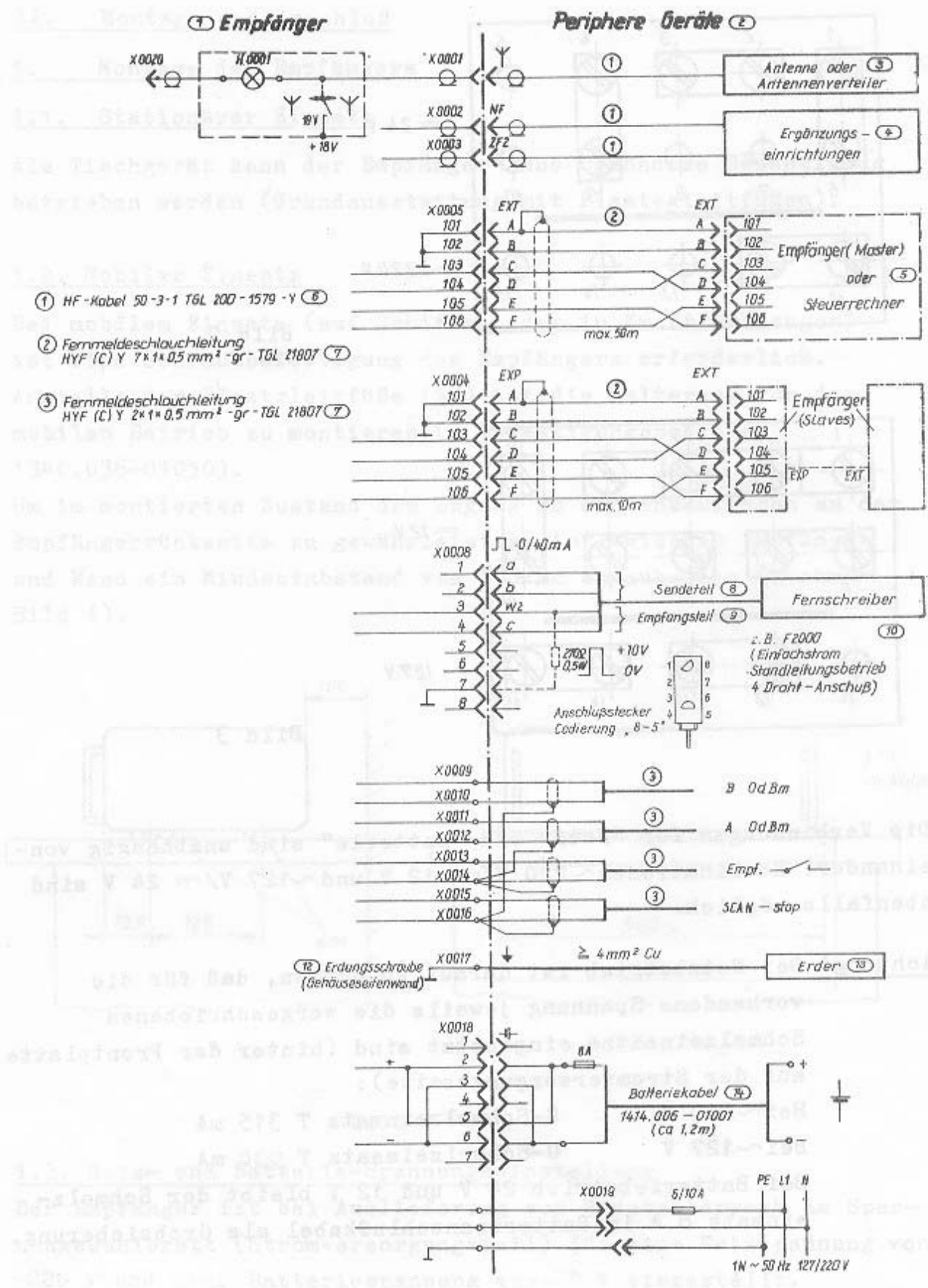
Anschlußplan 1340.042-00001 Ap
