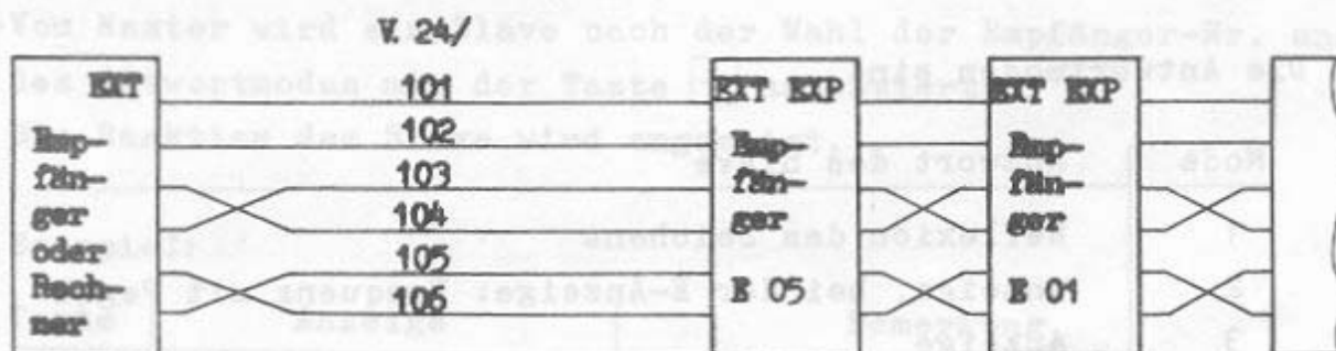
Zusammenschaltung ohne Modem
